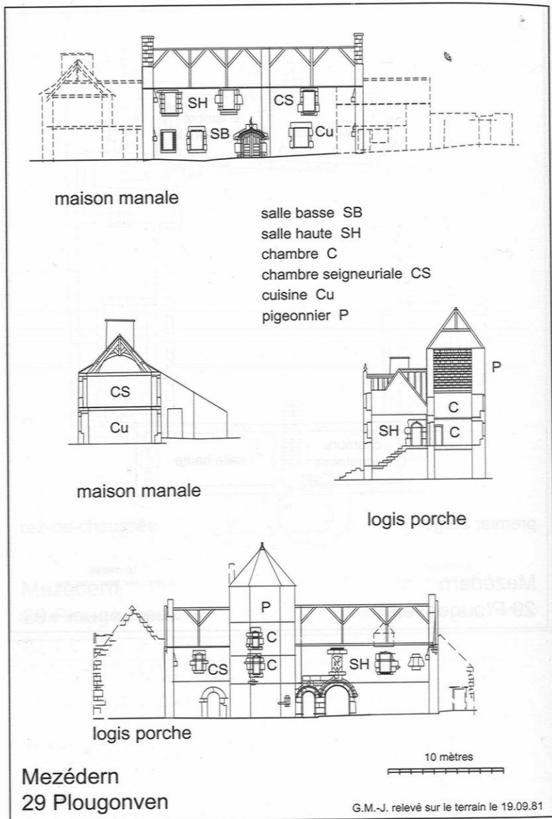
Figure 19. – Mezédern : coupes de la maison manale et du logis-porche Relevé et dessin : Gwyn Meirion-Jones
